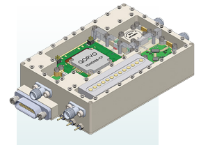
TxRx Modules
